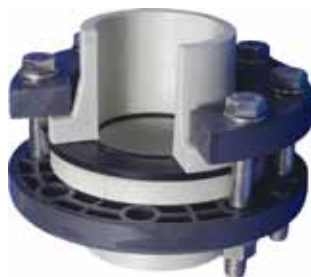
GSTP stålførsterket profilgummipakning tilpasset plastrørssystemer
