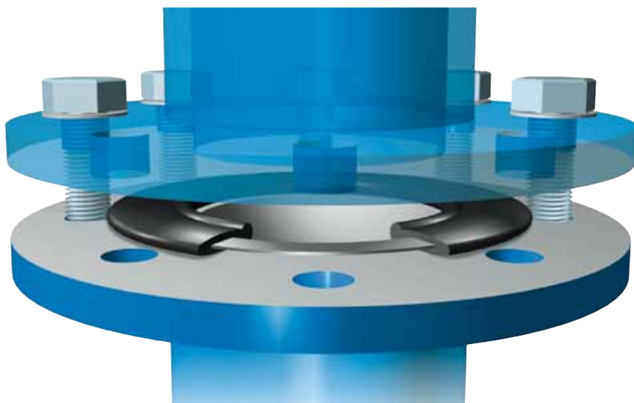
GSTP stålførsterket profilgummipakning tilpasset plastrørssystemer
